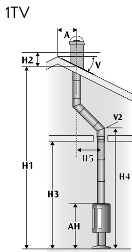
Górny wylot spalin, częściowo izolowany, z przesunięciem.
