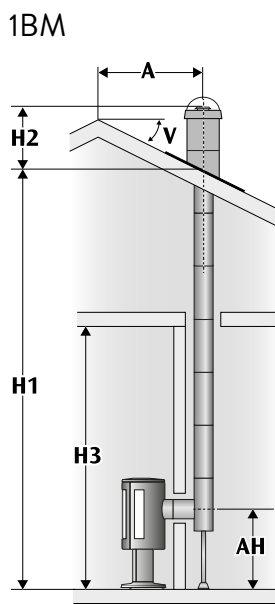
Tylny wylot spalin przez ścianę dachową, całkowicie izolowany.
