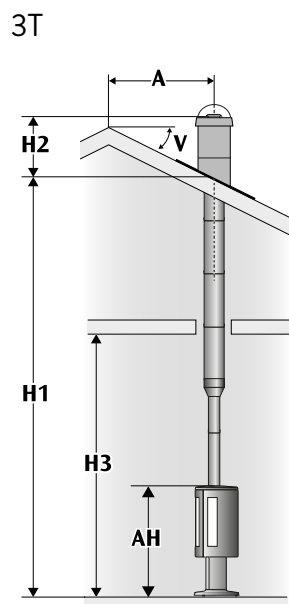
Górny wylot spalin, nieizolowany odcinek początkowy.
