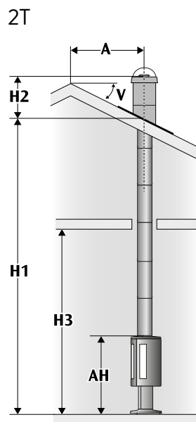
Górny wylot spalin, całkowicie izolowany.
