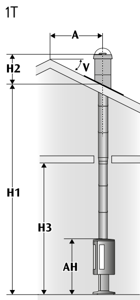
Górny wylot spalin, częściowo izolowany odcinek początkowy.
