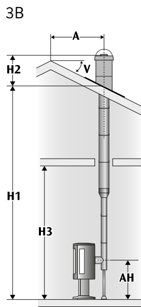
Tylny wylot spalin, nieizolowany odcinek początkowy.
