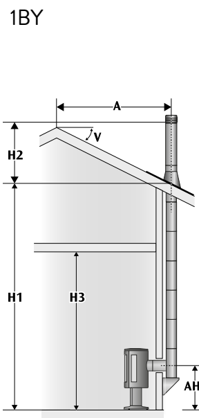
Tylny wylot spalin przez ścianę zewnętrzną, całkowicie izolowany.
