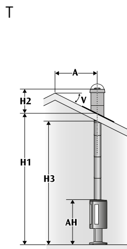
Górny wylot spalin, częściowo izolowany.
