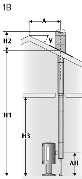
Tylny wylot spalin, częściowo izolowany odcinek początkowy.
