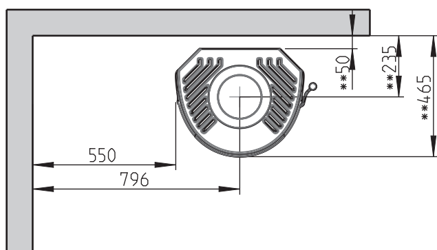
Ściana palna:
