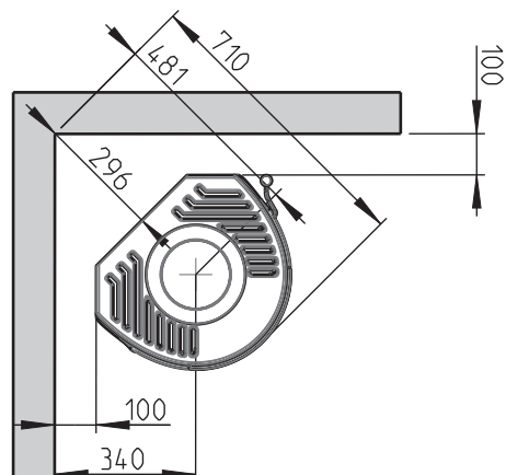
Ściana palna:
