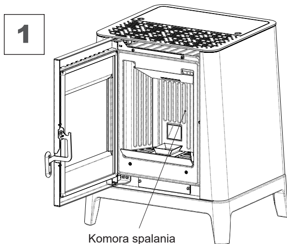
Komora spalania
